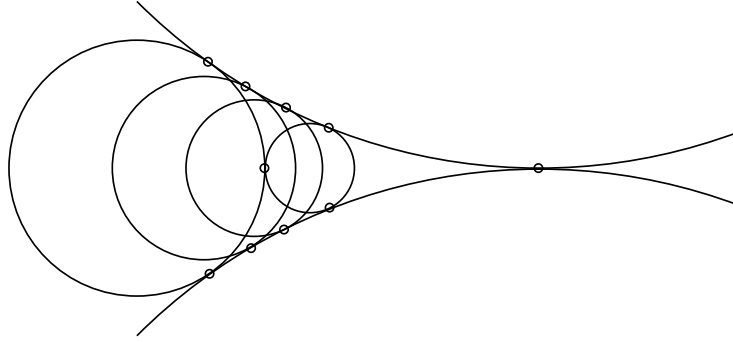
4. ábra. n kör lap 2n - 2 érintést határozhat meg.
