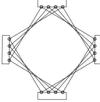
3. ábra. n konvex sokszög meghatározhat \Omega(n^2) érintést.
